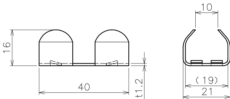
ロープクランプ
