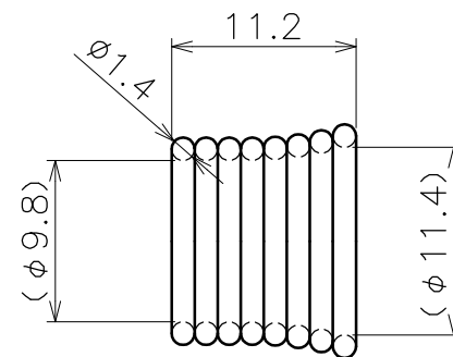
バネ S=2:1
